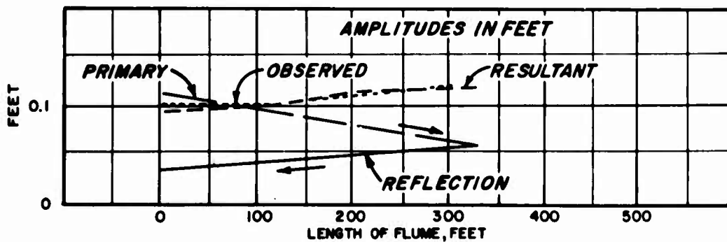
Fig. II-4. Vicksburg salinity flume tides
