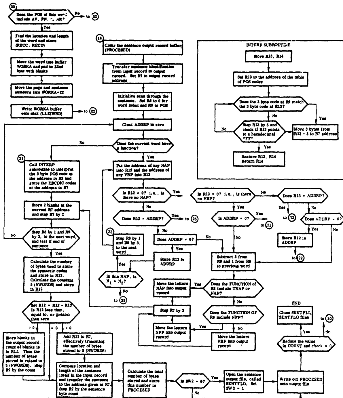
Fig. 3 BPHRAS Flow Diagram (Cont.)
