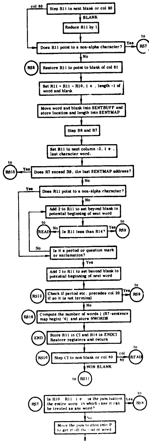
Fig. 7 LLEMREAD Subroutine (Cont.)
