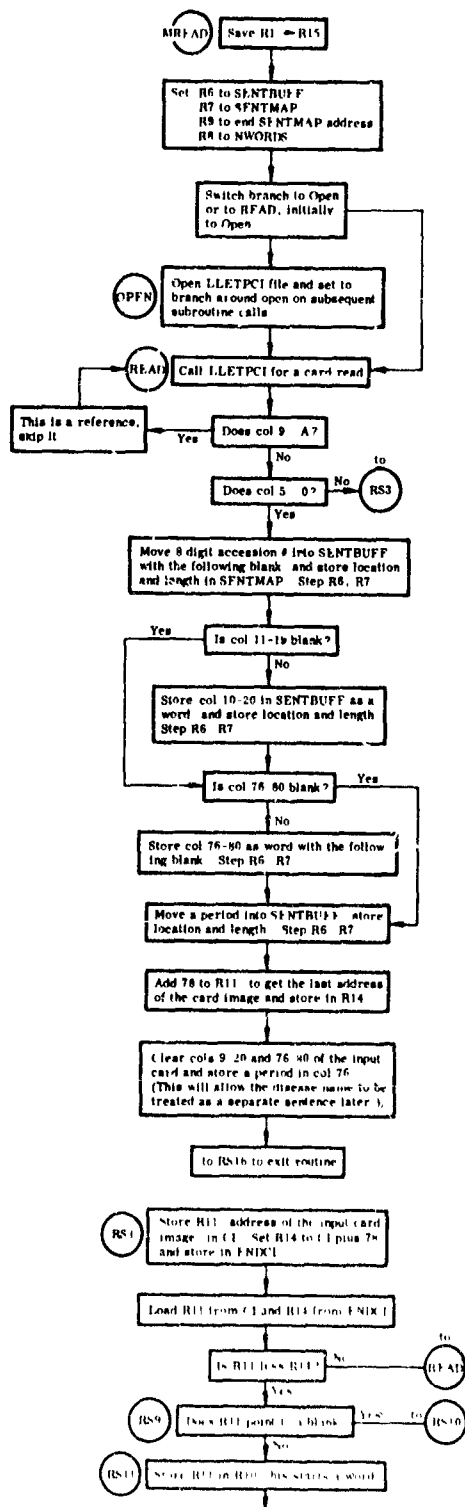
Fig. 7 LLEMREAD Subroutine
