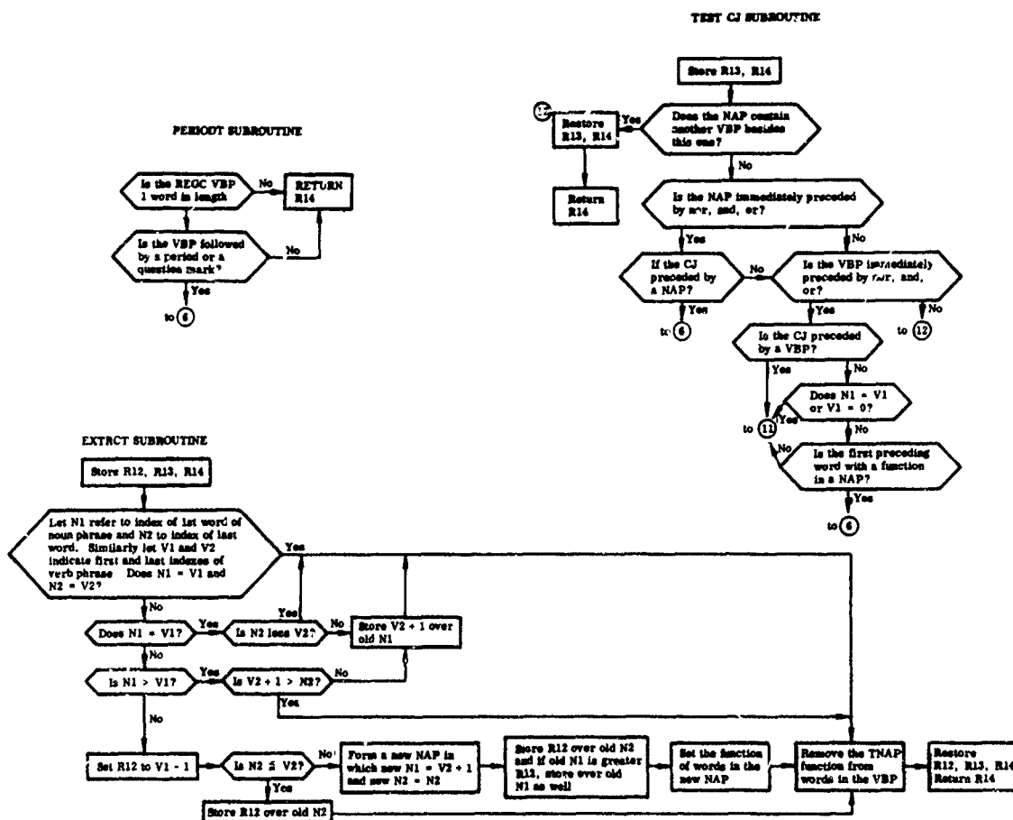
Fig. 3 BPHRAS Flow Diagram (Cont.)
