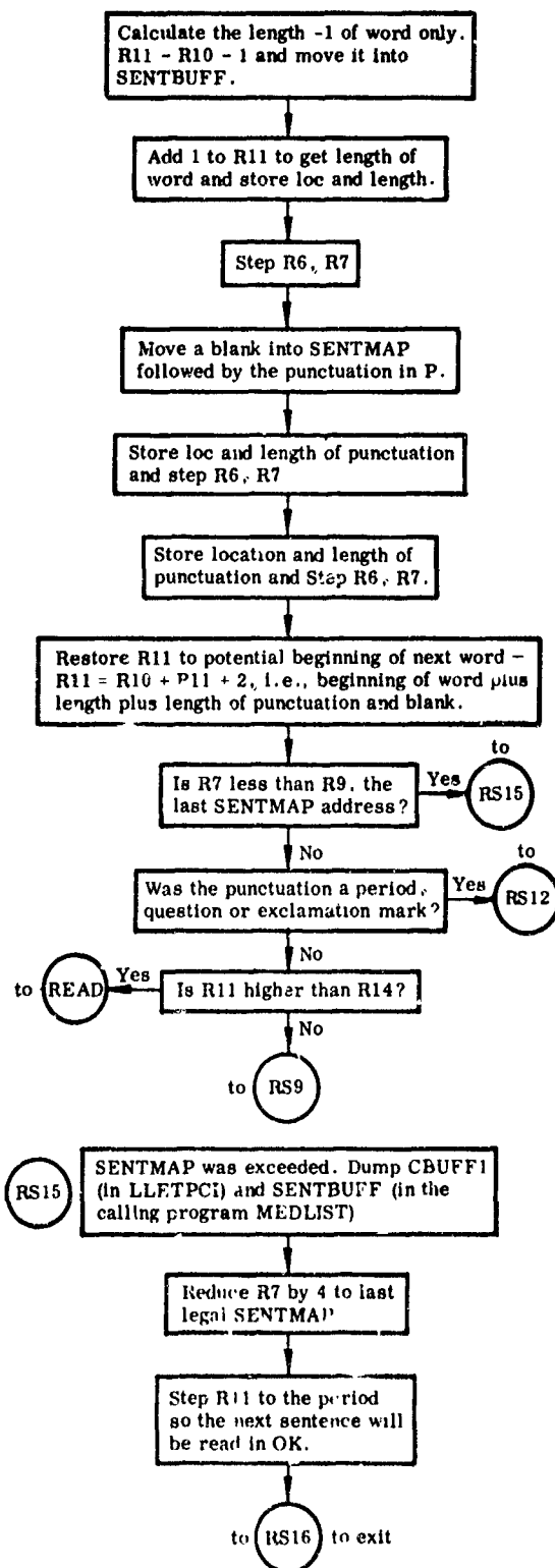
Fig. 7 LLEMREAD Subroutine (Cont.)
