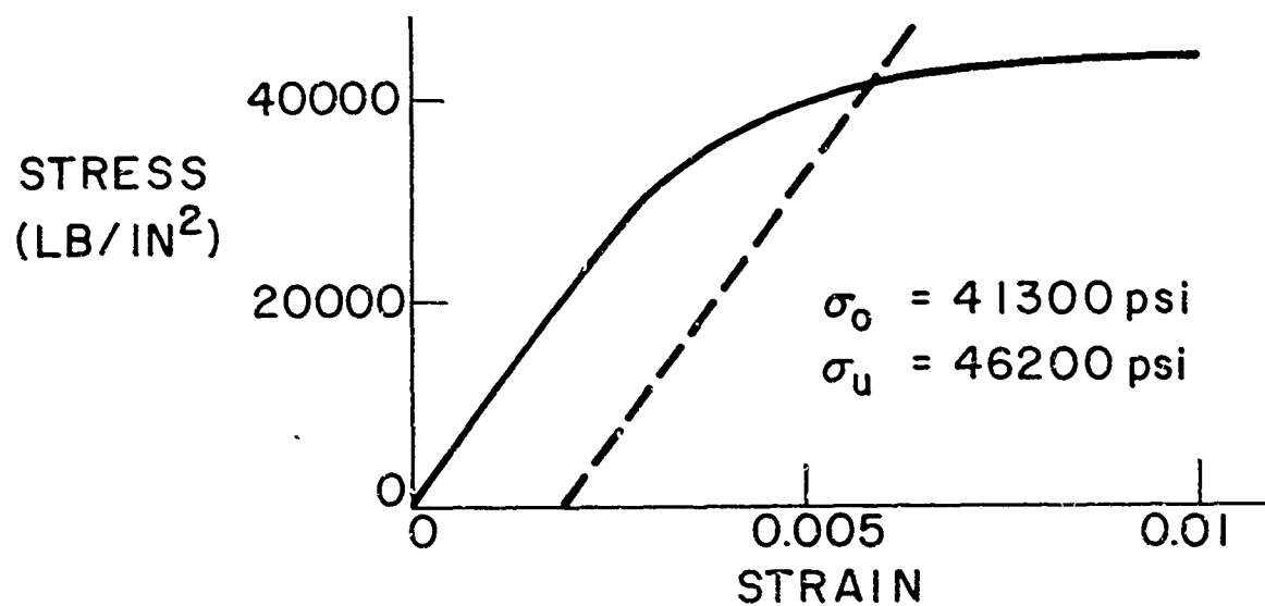
(b) ALUMINUM 6061-T6
