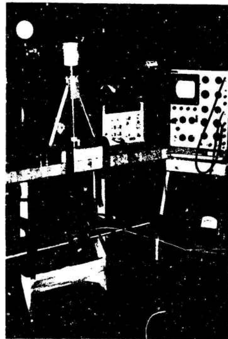
FIG. 7 ASSEMBLED TEST APPARATUS
