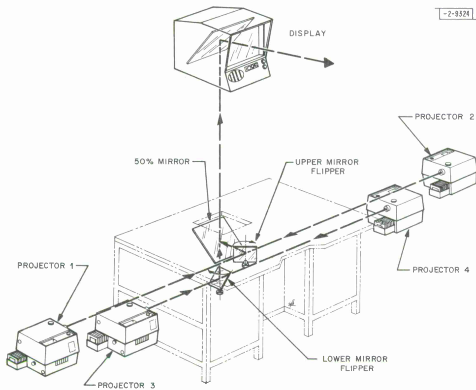
Fig. 2. LTS-1 (optics).
