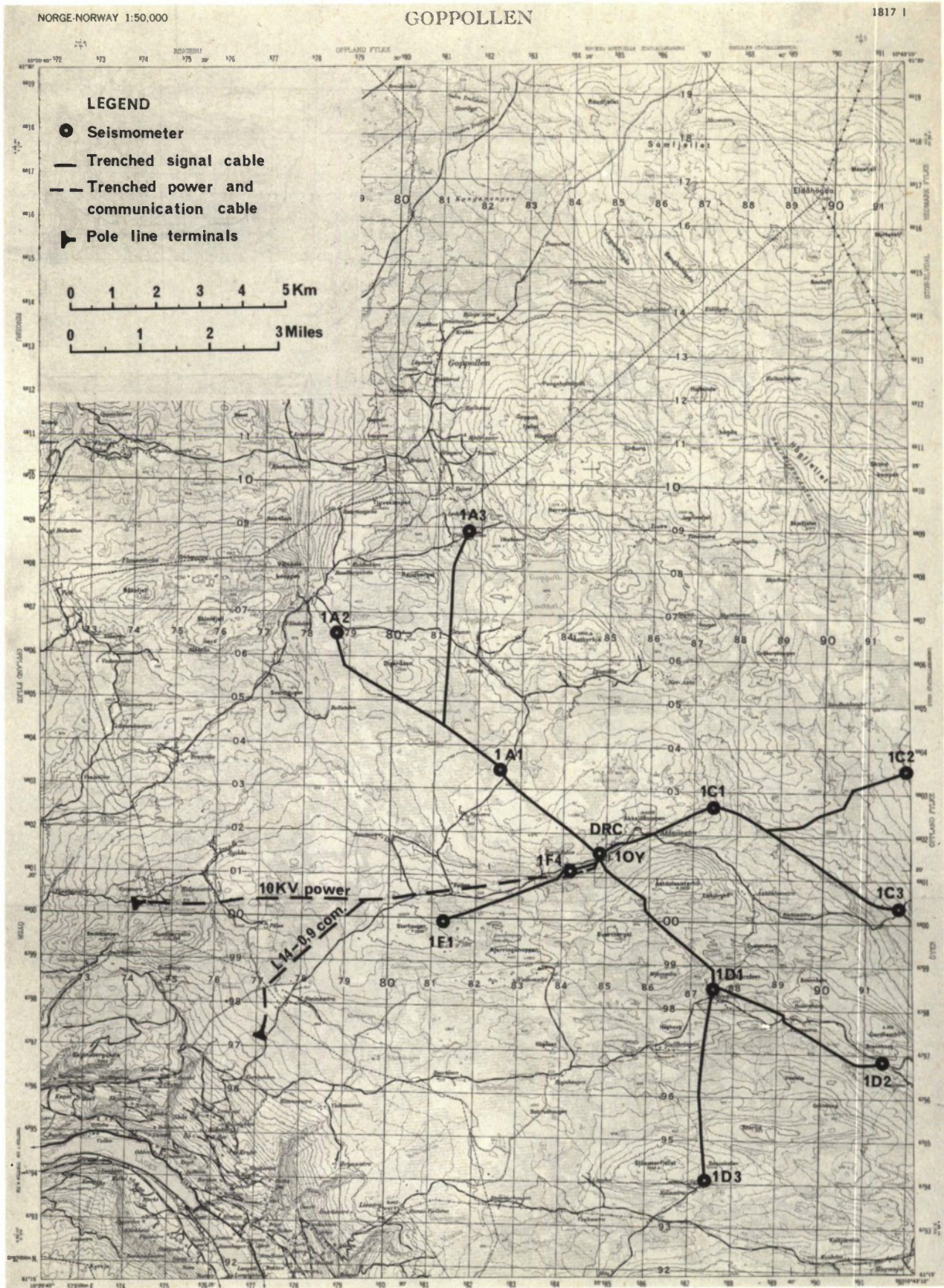
Figure 2.14 Oyer SP subarray, layout
