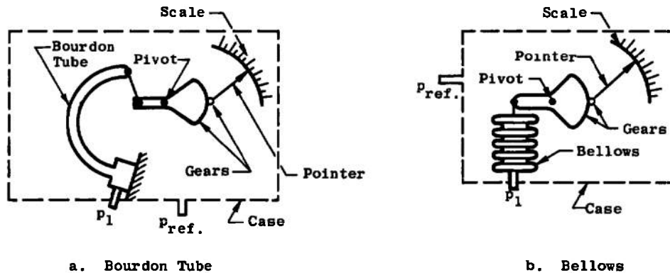
Fig. 81 Bourdon Tube Gages
