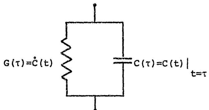
Adjoint Network, N
