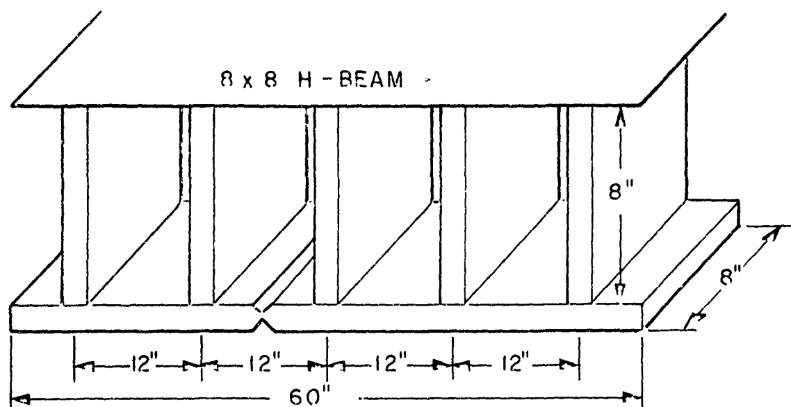
b. RIGID END SPECIMENS (NO. SR-MS-1,2; SR-80-1,2)
