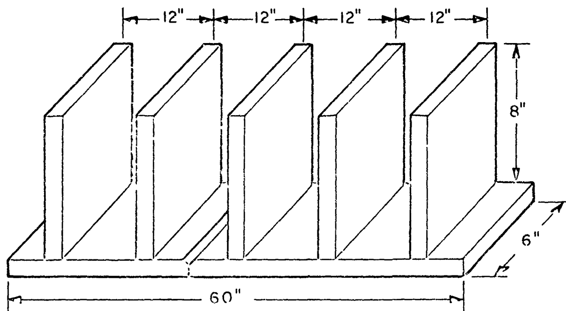
a. FREE END SPECIMENS (NO. SF-MS-1,2)
