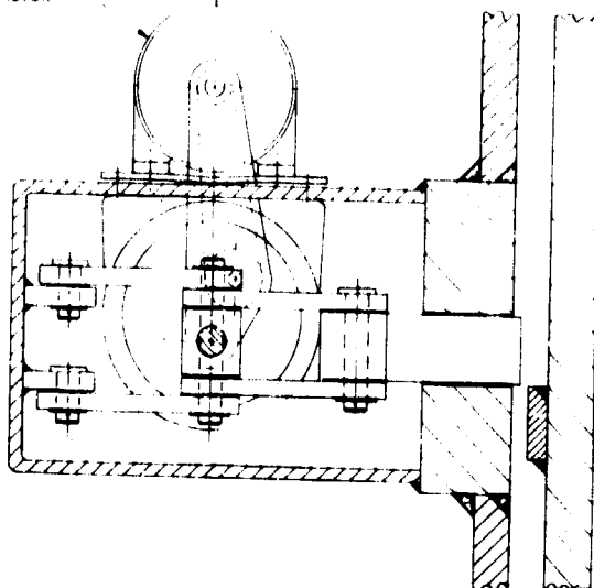
SECT 2-E SCALE: 3"=1'-0"
