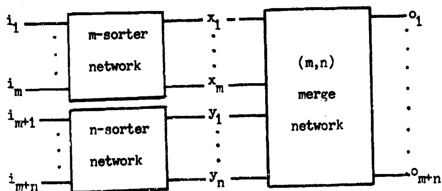
Fig. 4. (m+n) -sorter network T .
