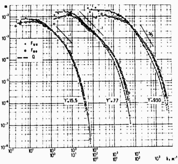
FIGURE 9 - SPECTRES DE VITESSE ET DE TEMPERATURE.
