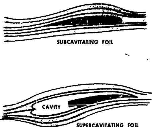
Fig. 14 - Cavitating foils
