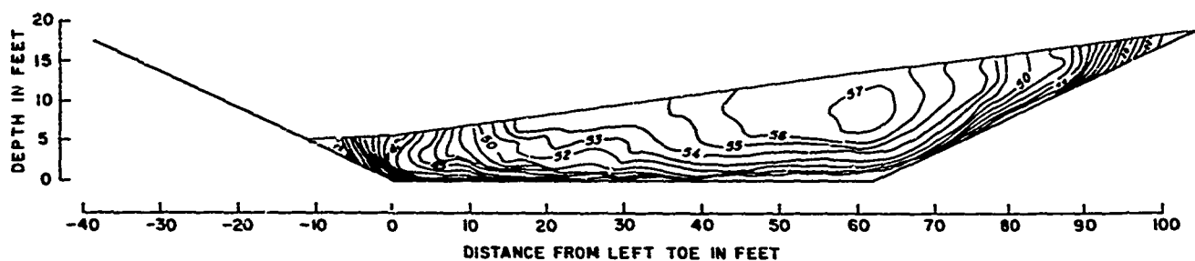
STA 22+50
