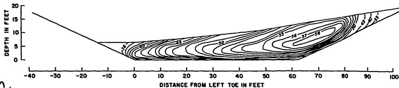
STA 34+00
