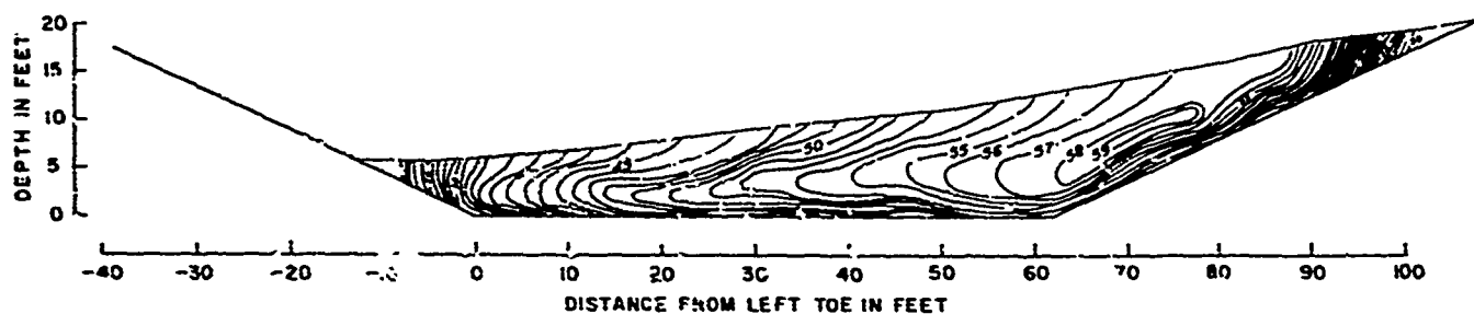
STA 33+00
