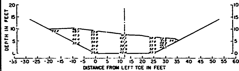
STA. 280+00
