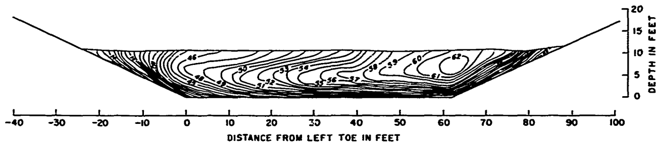
STA 49+00
