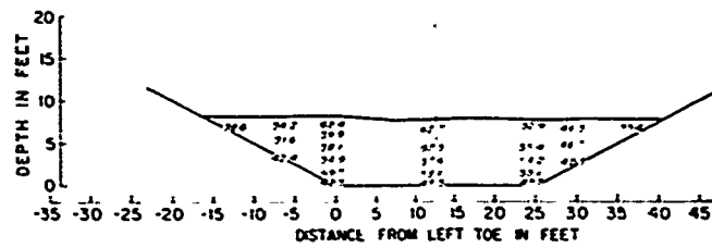
T.S. STA. 276+07.30
