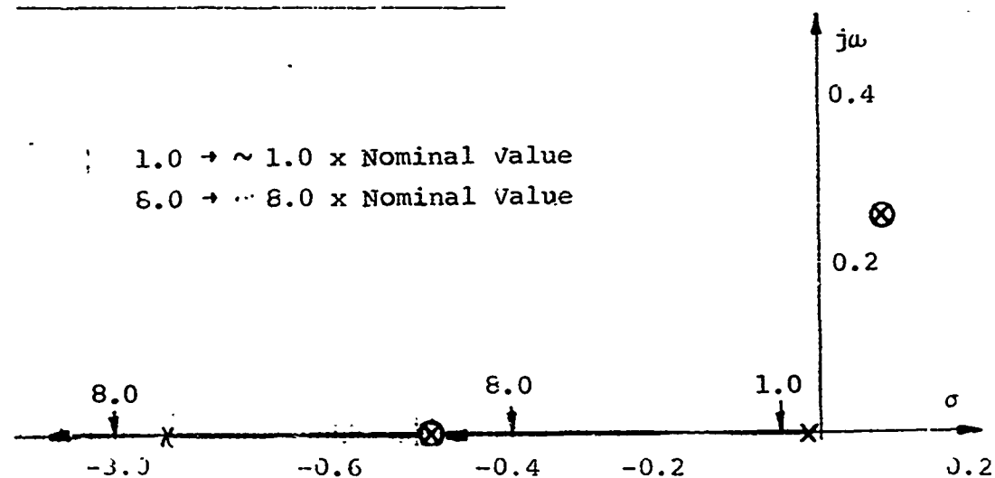
Figure 25. Hover Longitudinal M_u and Z_w Root Loci.
