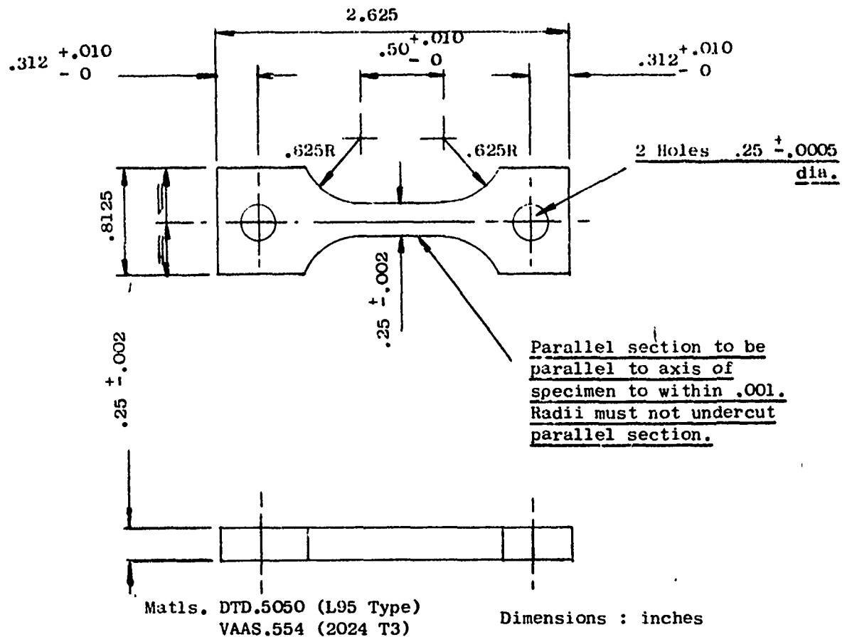
Fig. III : TENSILE TEST SPECIMEN
