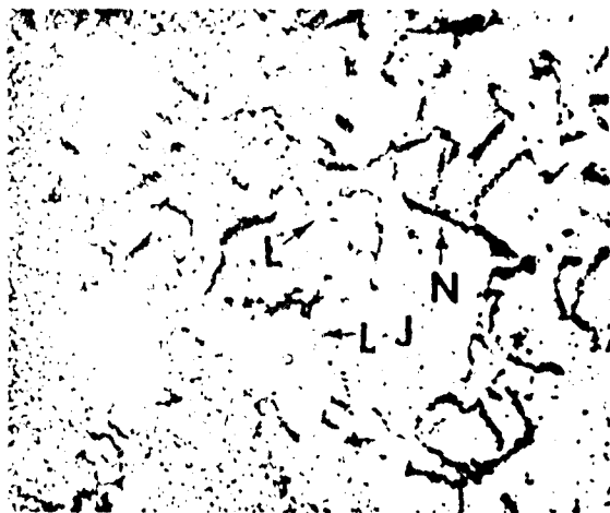
(422)
