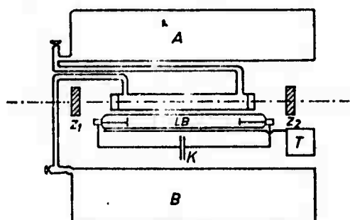
Fig. 1. Laser schematic
