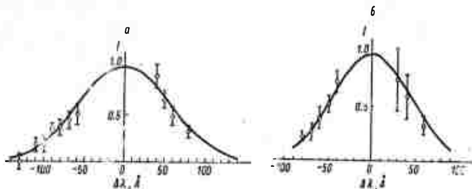
Fig. 2. Laser scatter spectra a- 4.5 ka; b- 9 ka.
