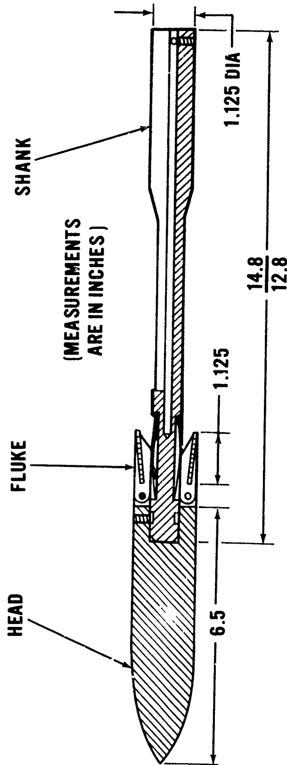
Fig. 45. Projectile.
