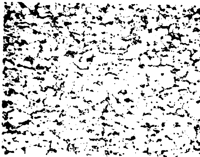
(d) Alloy 4. Ti-2.3Al-11.8Ga-1Mo-0.5Si, 1000X
