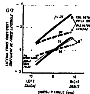
Fig 6. FENESTRON THRUST VS SIDESLIP (WIND TUNNEL TESTS) POL JEE FENESTRON EN FONCTION DU DERAPAGE (RESULTATS SOUFFLERIE)
