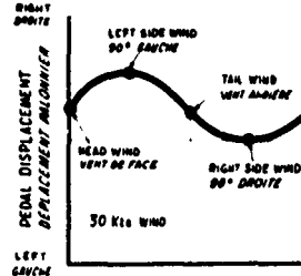
Fig 11. PEDAL DISPLACEMENT VS WIND HEADING IN HOVER DEPLACEMENT PALONNIER EN FONCTION DES CAPS AU VENT
