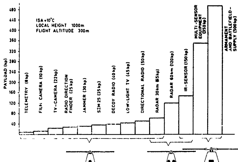
Fig. 19 Payload spectrum
