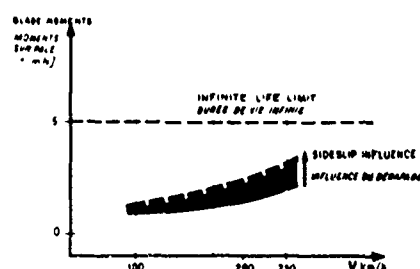
Fig 13. INFLUENCE OF SPEED AND SIDESLIP ON STRESSES EVOLUTION DES CONTRAINTES AVEC LA VITESSE
