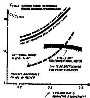
Fig 8. COMPARISON OF THRUST POSSIBILITIES OF CONVENTIONAL ROTOR AND FENESTRON COMPARAISON DES POSSIBILITES EN POUSSEE DU ROTOR CLASSIQUE ET DU FENESTRON
