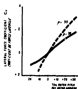
Fig 7. FENESTRON THRUST VS PITCH (WIND TUNNEL TESTS) POUSSEE FENESTRON EN FONCTION DU PAS (RESULTATS SOUFFLERIE)
