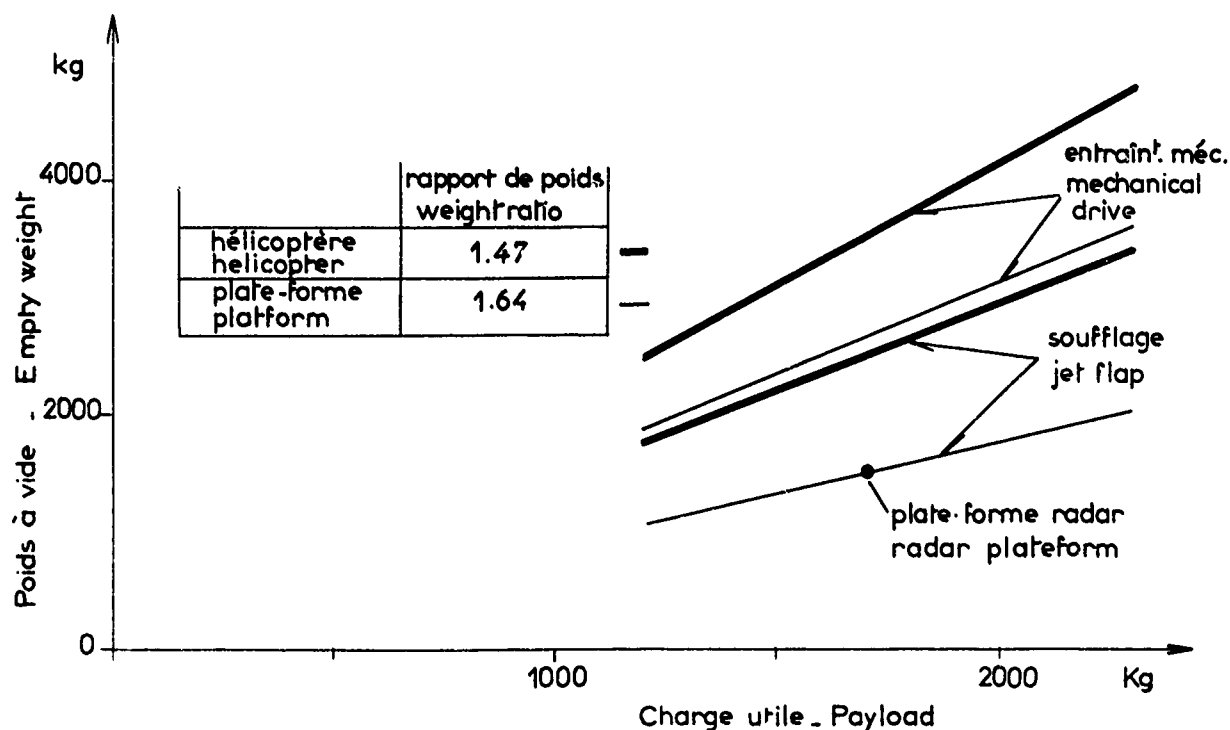
Fig.10 Comparison between shaft driven and jet-flap helicopters Comparaison entre les hélicoptères mécaniques et a volets fluides
