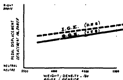
Fig 10. PEDAL DISPLACEMENT VS WEIGHT TO DENSITY RATIO IN HOVER DEPLACEMENT PALONNIER EN FONCTION DE LA MASSE REPUTEE EN STATIONNAIRE
