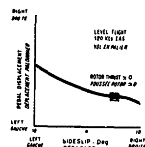
Fig 9. PEDAL DISPLACEMENT VS SIDESLIP DEPLACEMENT PALONNIER EN FONCTION DU DERAPAGE
