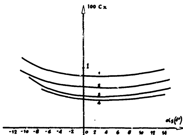
SA341 RECORD MESURES de TRAÎNÉ en SOUFFLERIE DRAG MEASUREMENTS IN WIND TUNNEL
