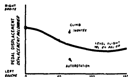
Fig 12. PEDAL DISPLACEMENT VS FORWARD SPEED DEPLACEMENT PALONNIER EN FONCTION DE LA VITESSE
