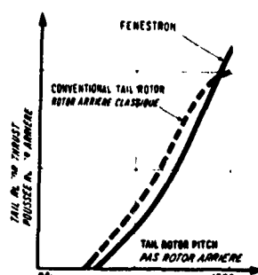
Fig 4. TAIL ROTOR THRUST VS PITCH IN HOVER POUSSEE ROTOR ANTICOUPEL EN STATIONNAIRE
