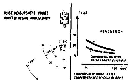
Fig 14. NOISE MEASUREMENTS ON FENESTRON MESURE DE BRUIT SUR FENESTRON
