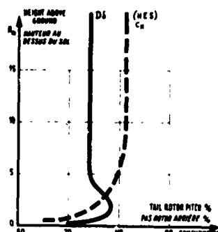
Fig 5. INFLUENCE OF GROUND ON FENESTRON INFLUENCE DU SOL SUR LE FENESTRON
