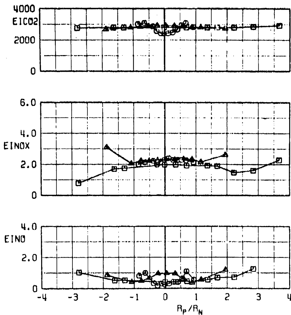
f. EICO_2 , EINO_x , and EINO versus R_p/R_N Fig. 17 Continued
