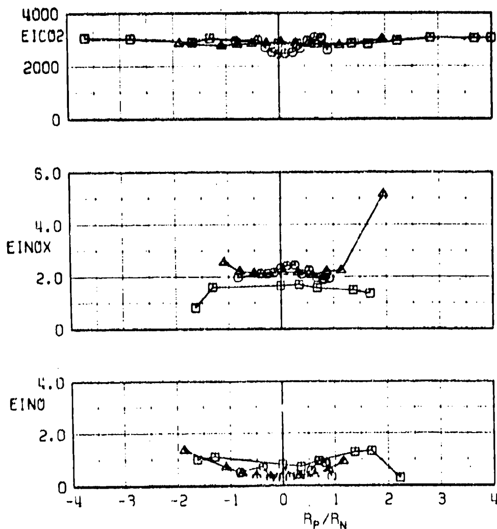
f. EICO_2 , EINO_x , and EINO versus R_p/R_N
