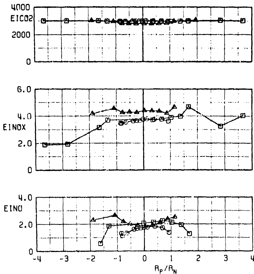
f. EICO_2 , EINO_x , and EINO versus R_p/R_N Fig. 14 Continued
