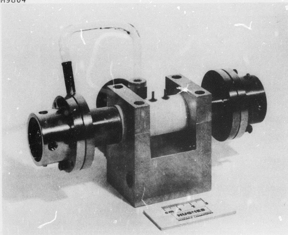
Fig. 4. Tunable laser.
