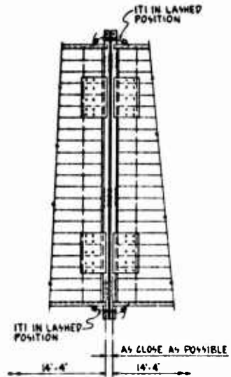
DET C (LASHING RAMP)
