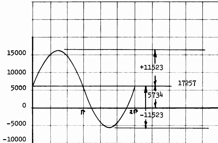
(a) ACTUAL OUT-OF-PLANE SHEAR LOAD
