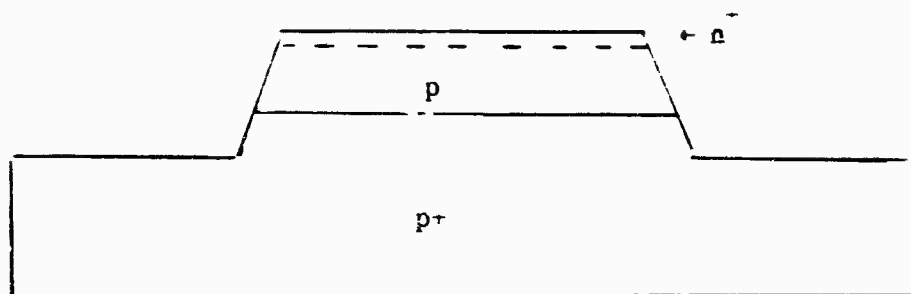
(a) Diffusion Photodiode
