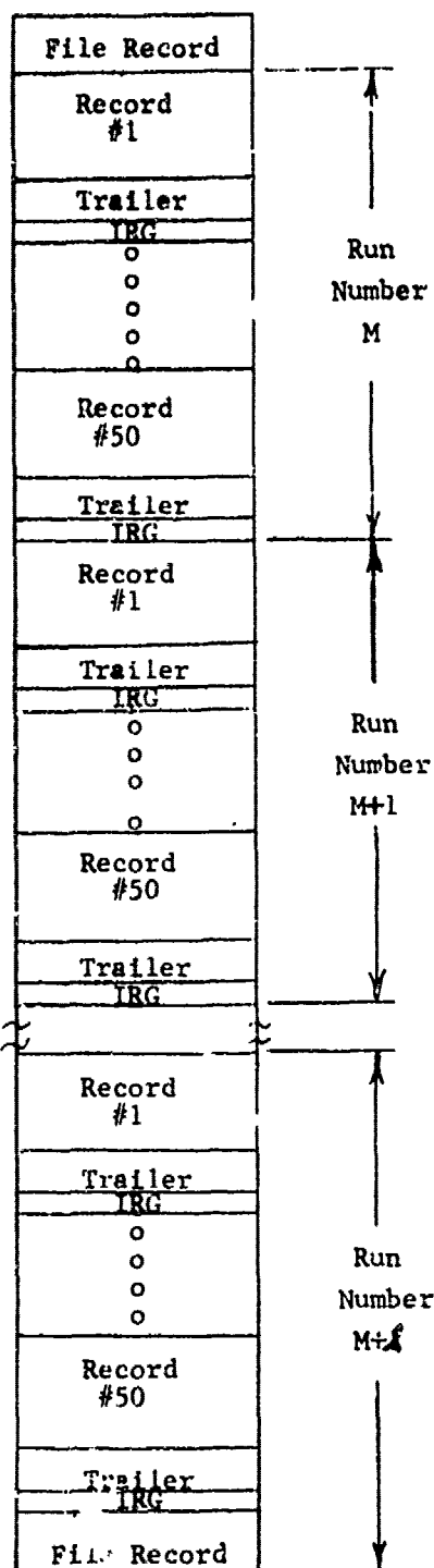
Fig. A-2 TAPE FORMAT
