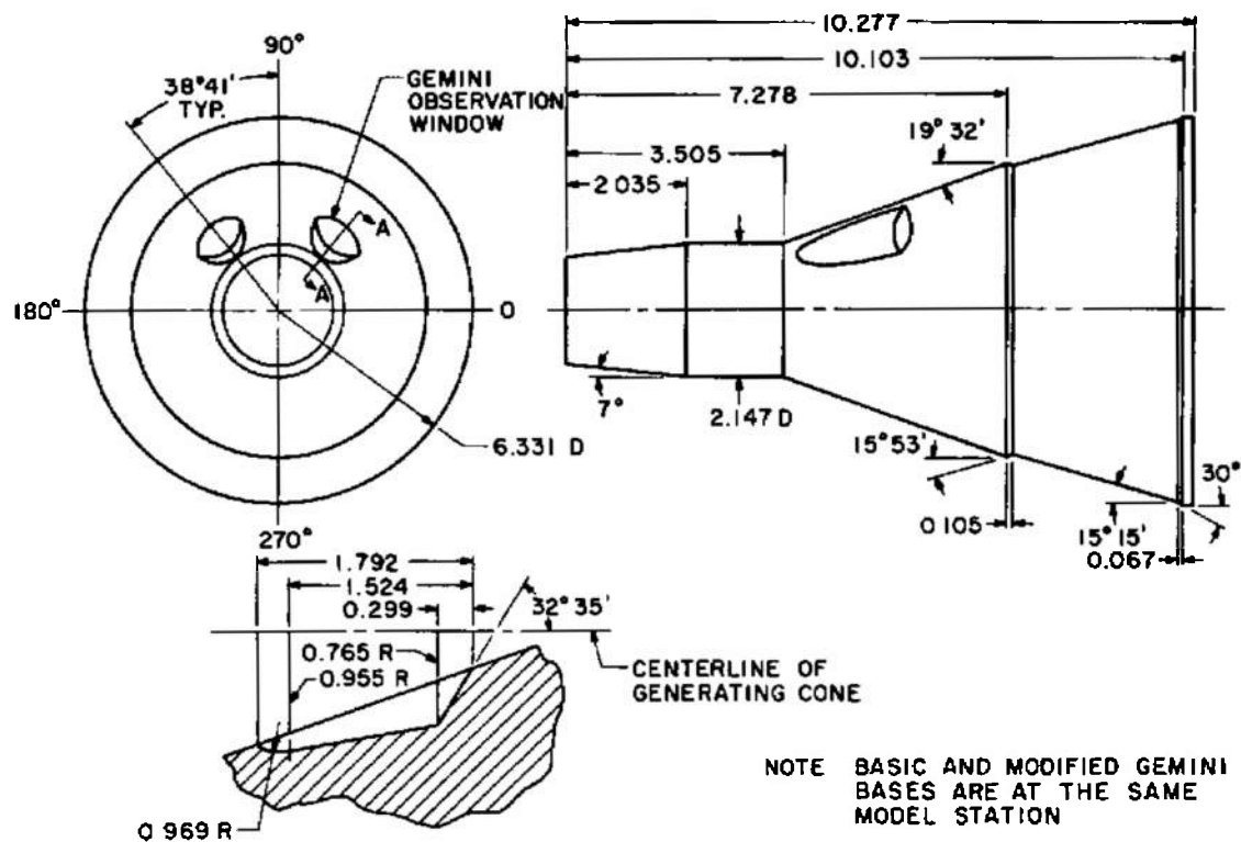
VIEW A-A
