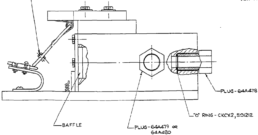
VIEW A-A
