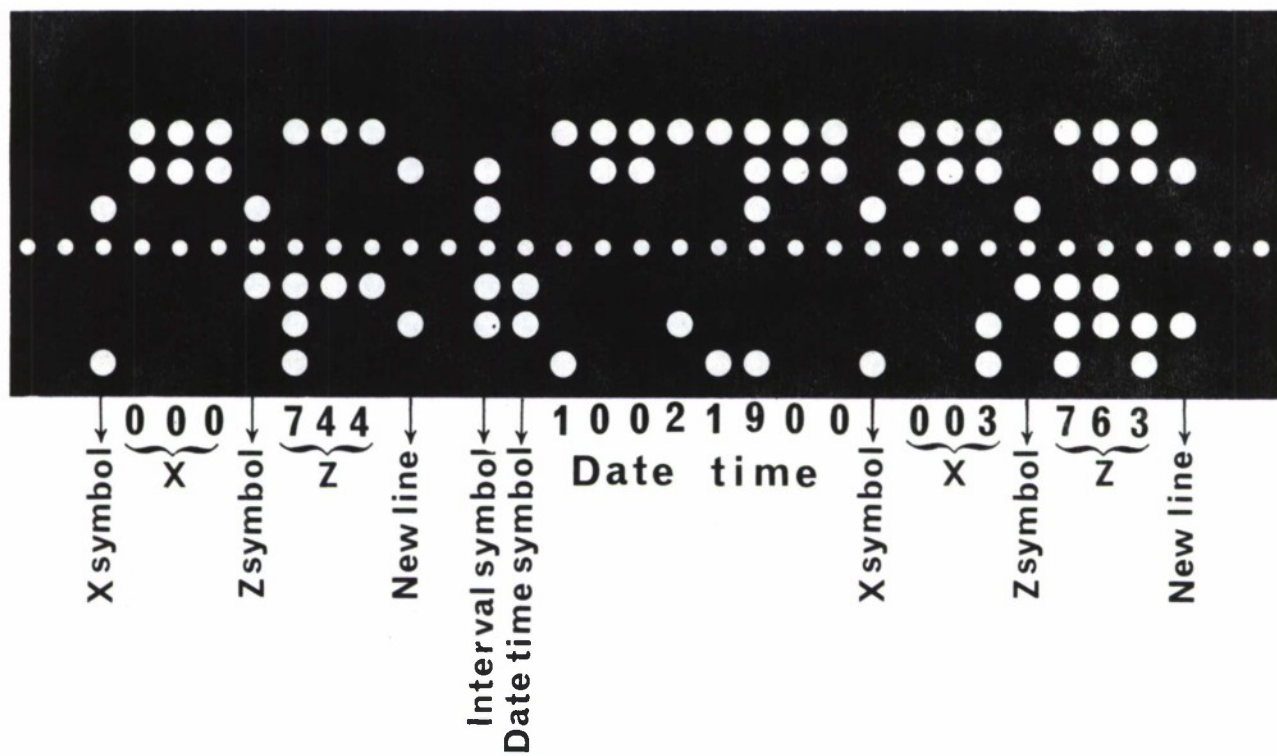
FIG. B.2 TAPE FORMAT
