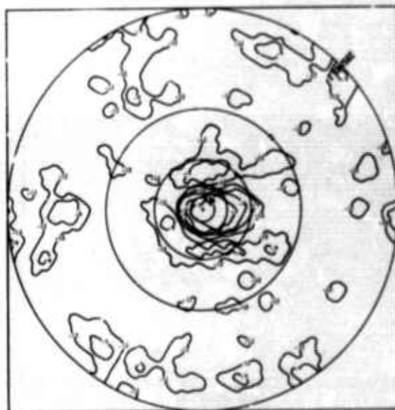
SUBARRAY C2
