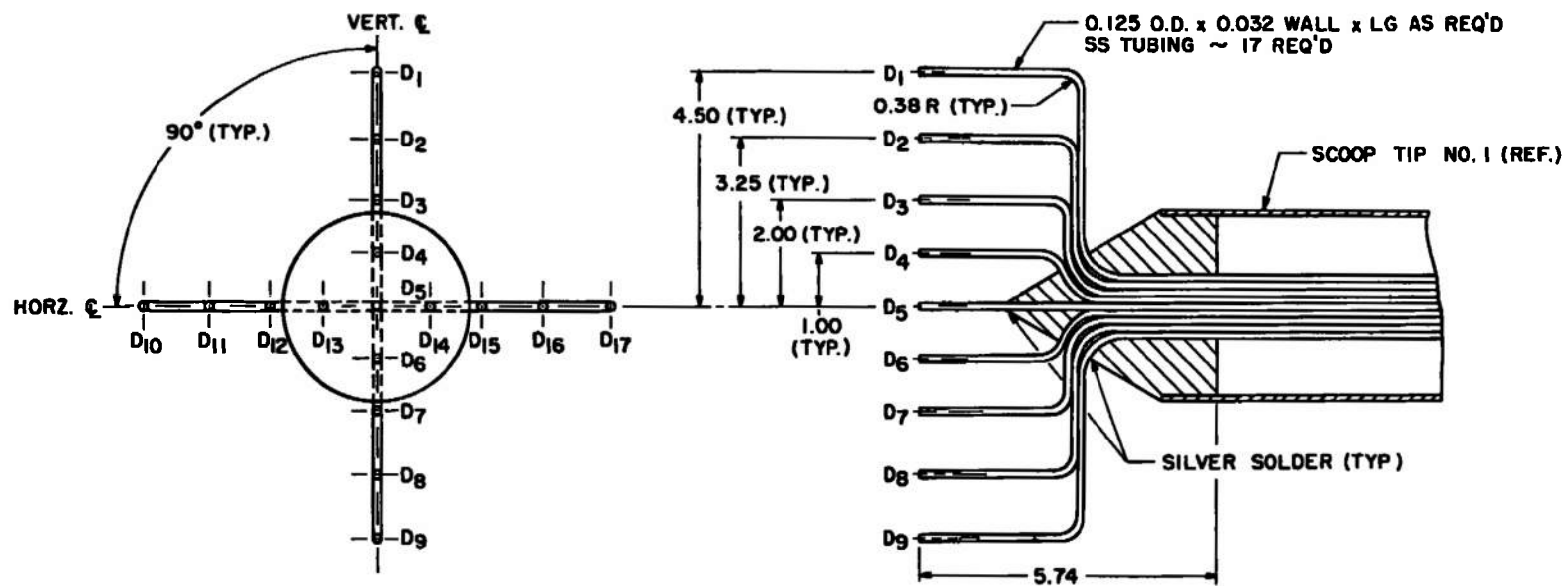
Fig. 6 Wake Rake
