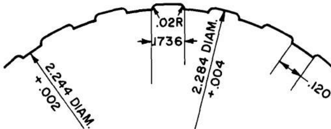
2.244 (57MM) RIFLING
