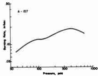
FIG. A-8. Burning Rate for Propellant A-157.
