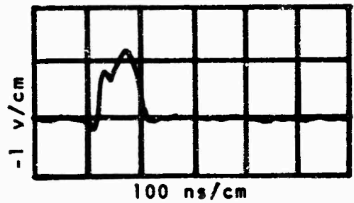
e) V_b=0 , Diodes In, V_x=75
