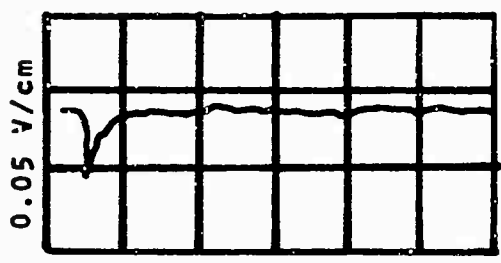
100 ns/cm b) V_{eb}=10.5, V_x=39
