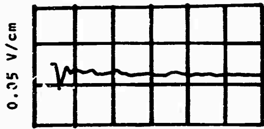
100 ns/cm b) V_b=1, V_x=20
