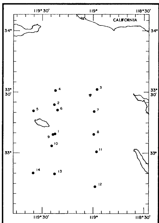
PLANKTON
