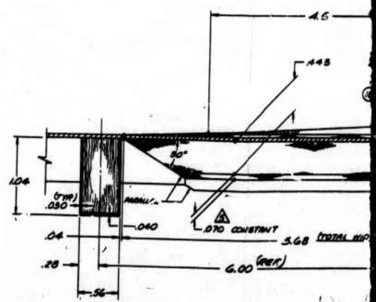
DETAIL 15 8 X 5 1/2 (ZONE G-H)
