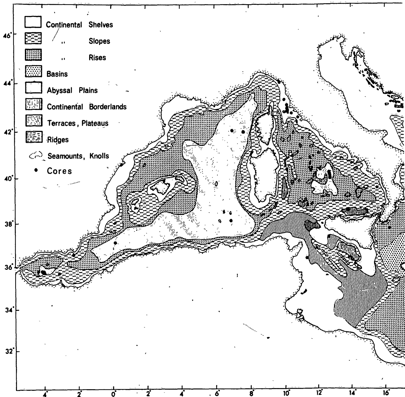
FIG. 4 MAJOR PHYSIOGRAPHIC REGIONS OF THE MED
