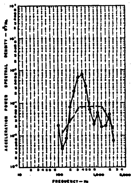
ACCELEROMETER - I
