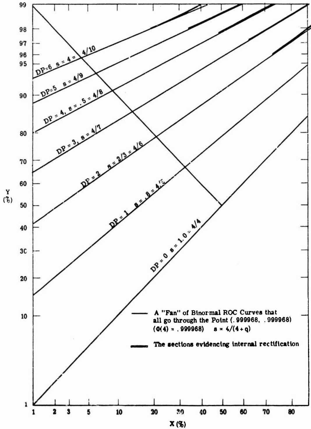
Fig. 7.14. A fan of binormal ROC curves
