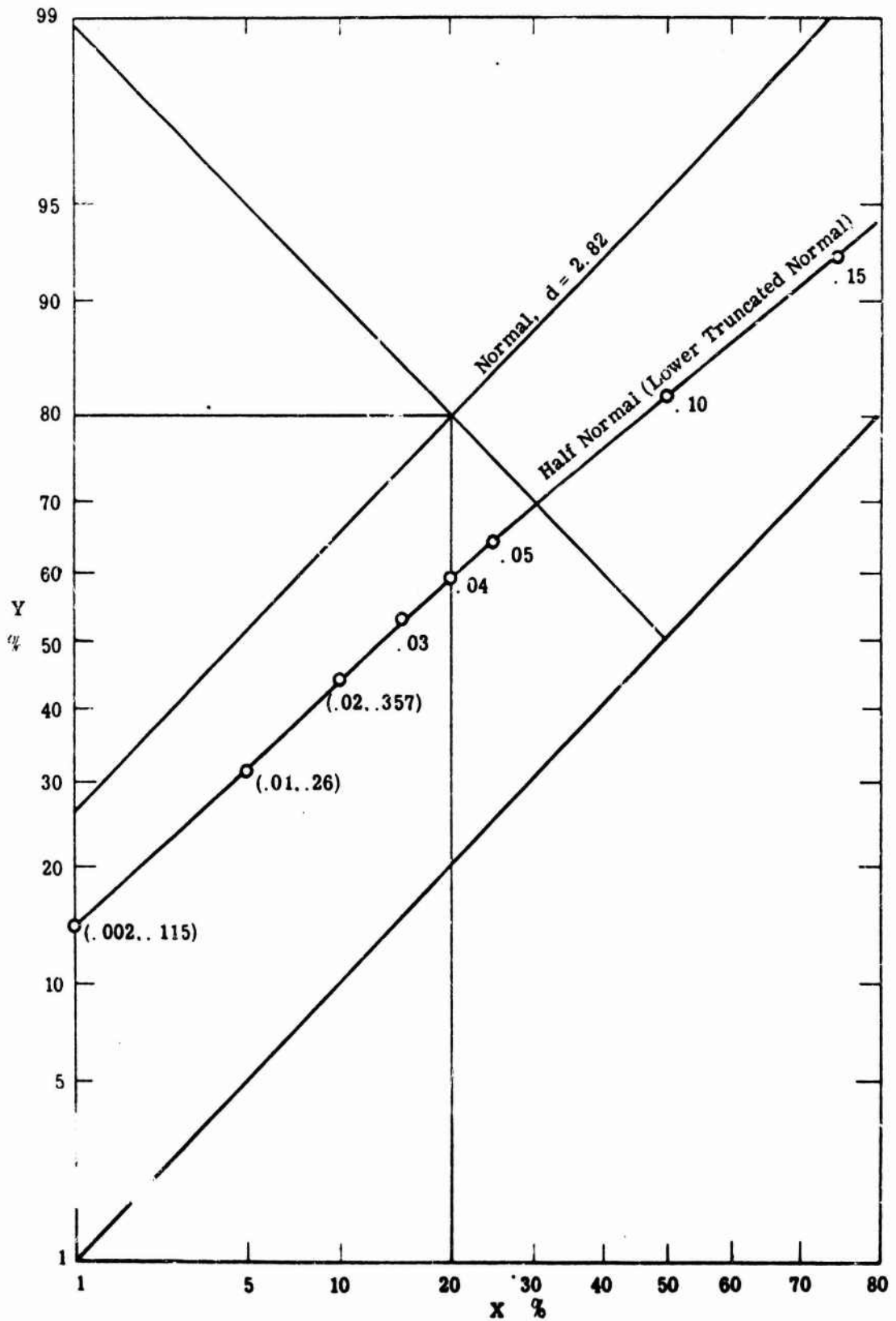
Fig. 3.3. Replot of Fig. 3.2
