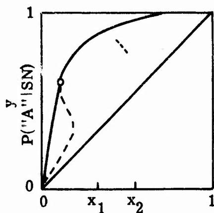
(d) Convex completion of (c)
