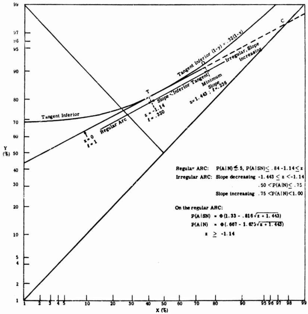
Fig. 7.6. Binormal ROC q = 2 s = .5
