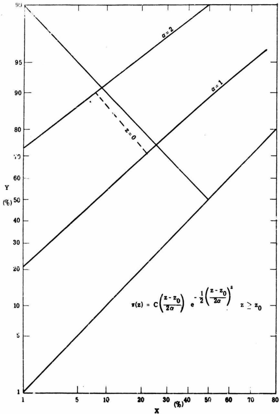
Fig. 9.4. H-type ROC, n = 1
