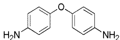
4,4'-oxydianiline
