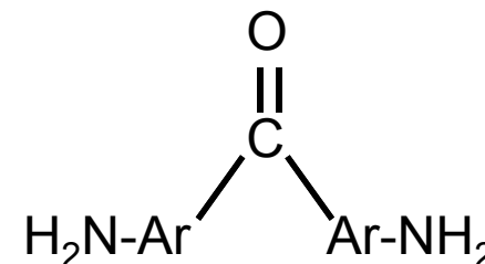
LARC-TPI
