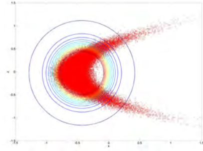
(d) (x, z) : upto 2^{nd} order moments
