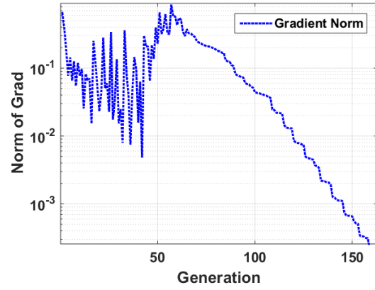
(b) 10-D Griewank
