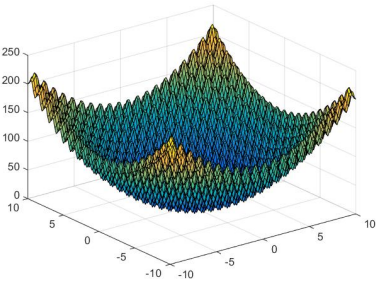
(d) Rastrigin
