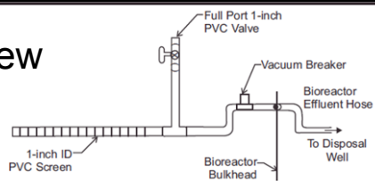
EFFLUENT DETAIL
