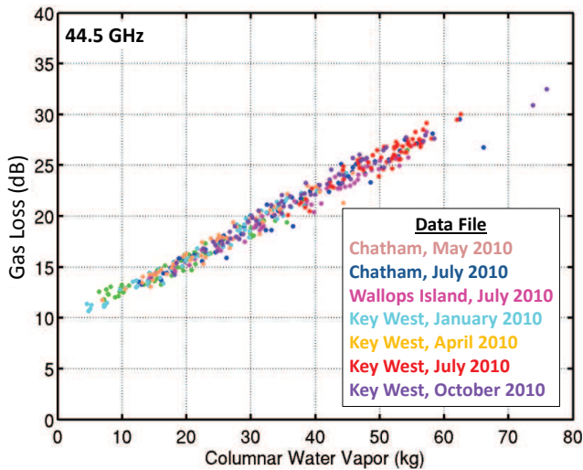
b. 44.5 GHz
