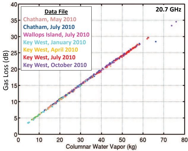
a. 20.7 GHz
