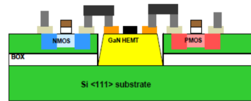
GaN HEMT/CMOS
