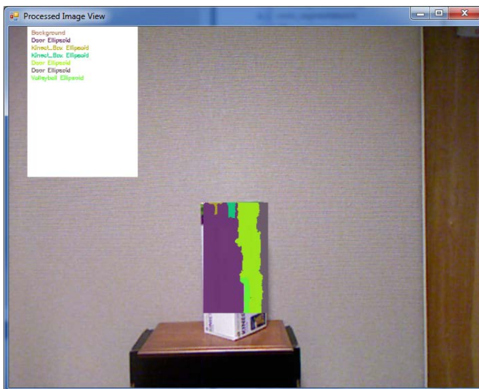
Fig. 111 Segmented ROI
