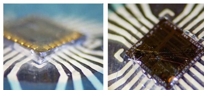
Fig. 4: 300um Die Delamination (L), 20um Materials Cracking (R)
