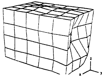
Mode 4 (1999.95 Hz)
