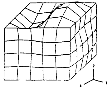
Mode 2 (1006 Hz)
