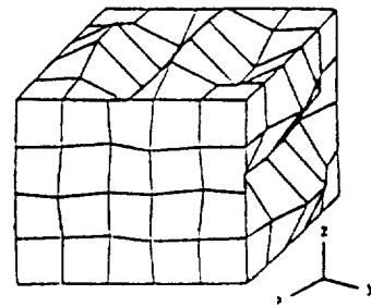
Mode 6 (2536 Hz)
