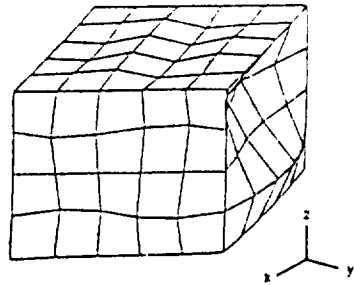
Mode 3 (1762 Hz)
