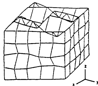
Mode 8 (3012 Hz)
