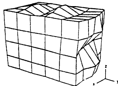
Mode 6 (2535.77 Hz)
