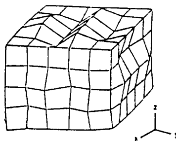
Mode 7 (2752 Hz)
