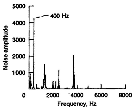
(d) Power spectrum for noise from microphone number 1.
